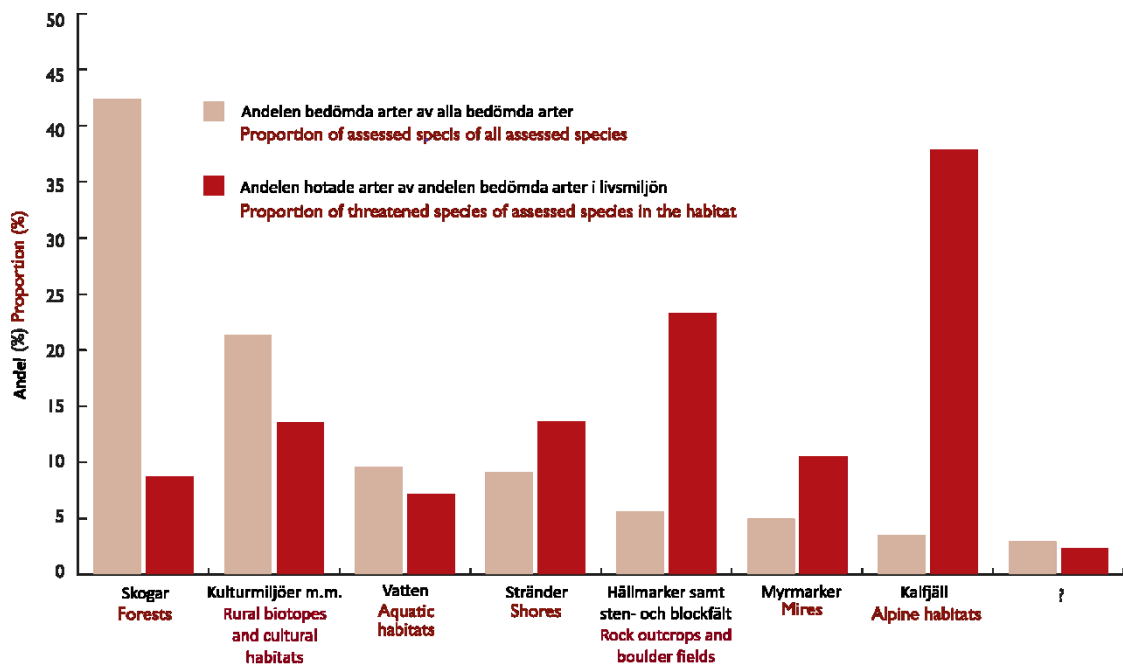
Figur 6. Fördelningen av bedömda och hotade arter enligt den huvudsakliga livsmiljön. Källa: Hyvärinen med flera 2019, s. 39.
