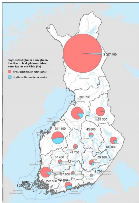
Figur 9. Skrydsfastigheter som staten besitter och skyddsområden som ägs av enskilda. I statliga naturskyddsområden har det föreslagits både naturskyddsområden som redan inrättats och områden som redan reserverats för naturskyddsändamål, men som ännu inte inrättats. Källa: Naturskydds- och ödemarksområden 2022, Forststyrelsens fastigheter 2021.
