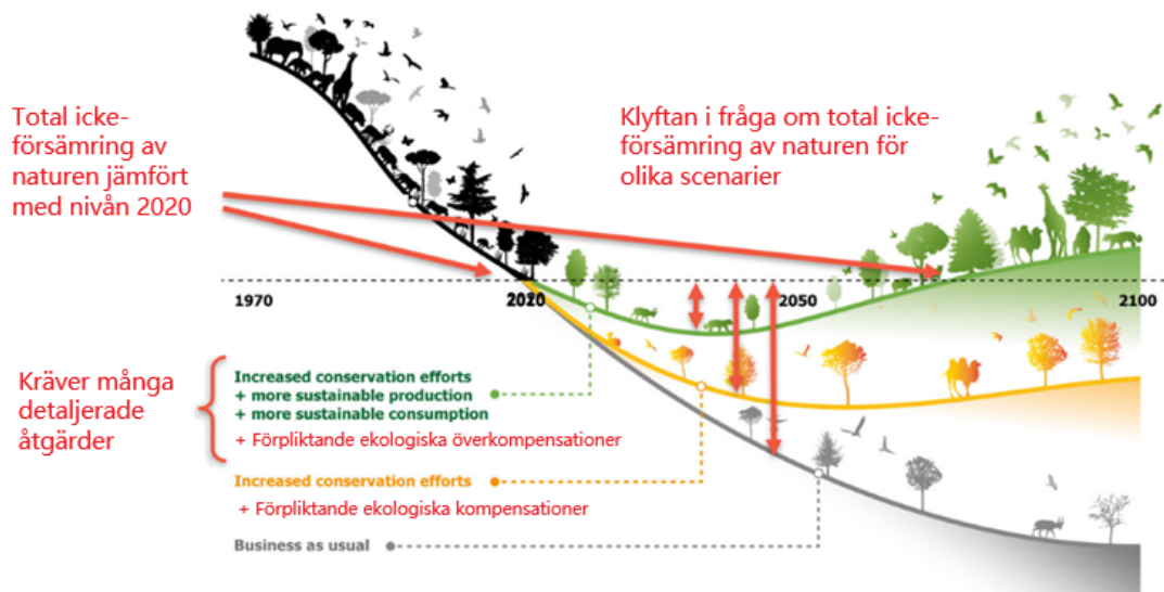
Figur 2. Total icke-försämring av naturen jämfört med nivån 2020 och klyftan i fråga om total icke-försämring för olika scenarier. Källa: Finlands Naturpanel 2021.
