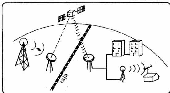
4. Yleisradiolähetyksen samanaikainen siirto välityssatelliitin (esimerkiksi ECS, Horizont) avulla edelleen lähetettäväksi kaapeliverkossa tai vapaasti etenevillä radioaalloilla.
