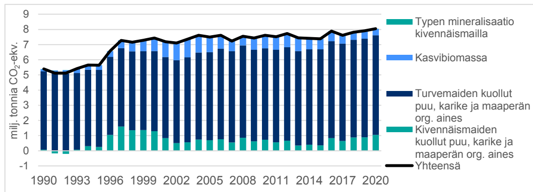
Kuva 16. Eri hiilivarastojen muutokset (negatiivinen merkitsee hiilivaraston kasvua, positiivinen vähenemistä) viljelysmaan maankäyttöluokassa ja hiilivarastomuutosten summana lasketut viljelysmaan kokonaispäästöt vuosina 1990–2020. Maatalousmaiden dityppioksidipäästöt (N 2 O) raportoidaan taakanjakosektorilla (pellonraivauksen dityppioksidipäästöjä lukuunottamatta), joten ne puuttuvat tästä kuvasta. Lähde: Tilastokeskus/Luonnonvarakeskus 2022.
