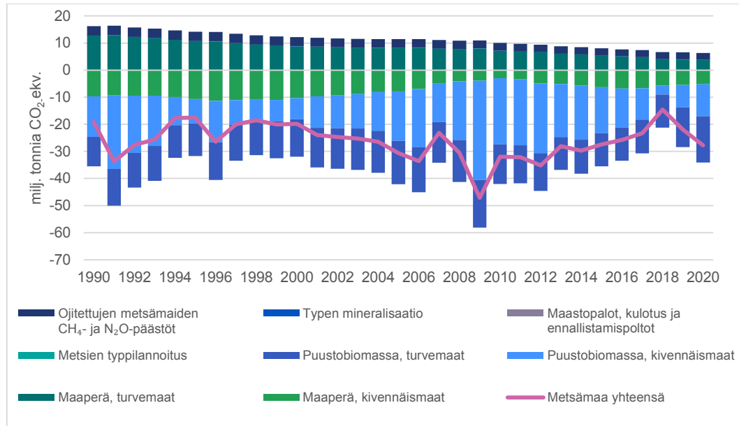
Kuva 15. Eri hiilivarastojen muutokset metsämaalla (negatiivinen merkitsee hiilivaraston kasvua, positiivinen vähenemistä) ja kasvihuonekaasupäästöt ojituksesta, typpilannoituksesta, maastopaloista ja typen mineralisaatiosta maaperän orgaanisen aineksen hajotessa ja kaikkien hiilivarastomuutosten ja päästöjen summa vuosina 1990–2020. Lähde: Tilastokeskus/Luonnonvarakeskus 2022.
