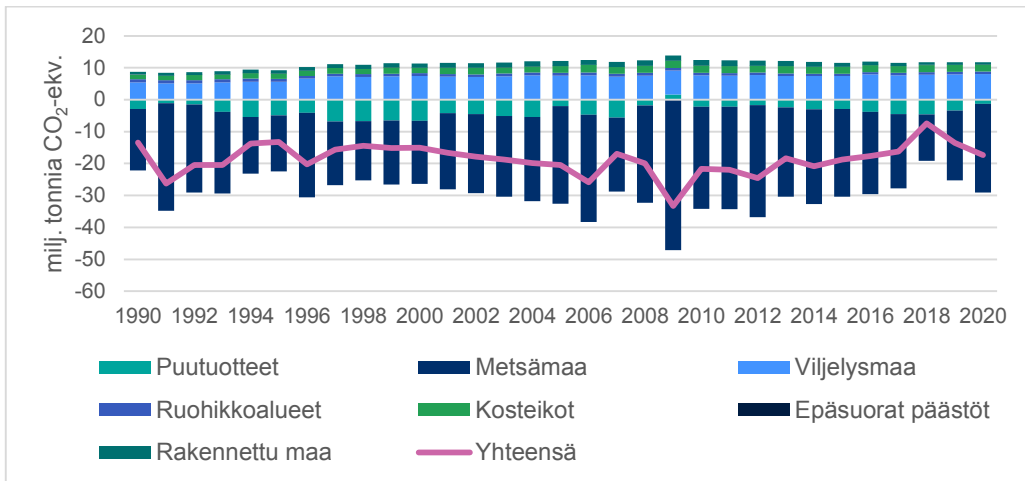
Kuva 12. Maankäyttöluokittaiset päästöjen ja poistumien summat maankäyttö, maankäytön muutokset ja metsätalous -sektorilla 1990–2020 (positiivinen tarkoittaa nettopäästöä ja negatiivinen nettopoistumaa). Maankäyttösektorin päästöjen ja poistumien summa on merkitty viivalla. Lähde: Tilastokeskus 2022a.
