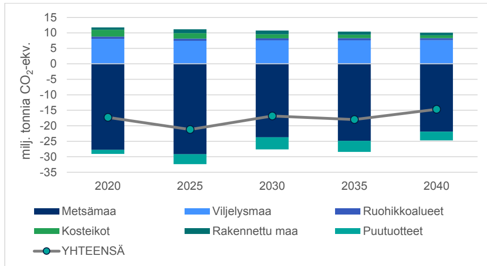
Taulukko 1. Maankäyttösektorin päästöt päästöluokittain perusskenaariossa, miljoonaa hiilidioksidiekvivalenttitonnia. Vuosi 2020 vastaa kasvihuonekaasuinventaarion arvoja AR5:n GWP-kertoimilla ja vuodet 2025–2040 ovat perusskenaarion tuloksia. Lähde: Luonnonvarakeskus 2022.
