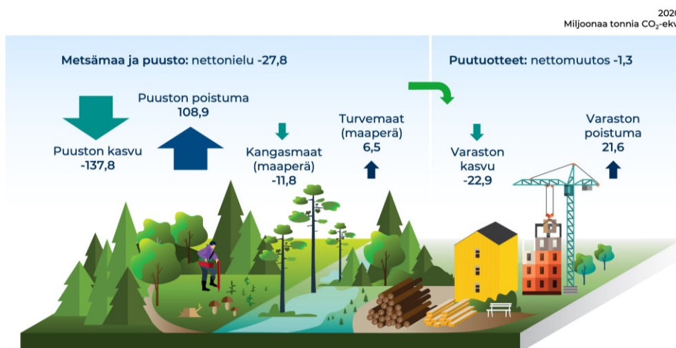
Kuva 6. Metsän ja puutuotteiden hiilitase vuonna 2020 (miljoonaa hiilidioksidiekvivalenttonnia). Lähde: Luonnonvarakeskus/Tilastokeskus 2022a.
