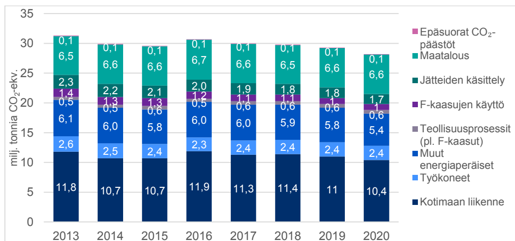
Kuva 11. Taakanajosektorin kasvihuonekaasupäästöt vuosina 2013–2020. Lähde: Tilastokes- kus 2022a.
