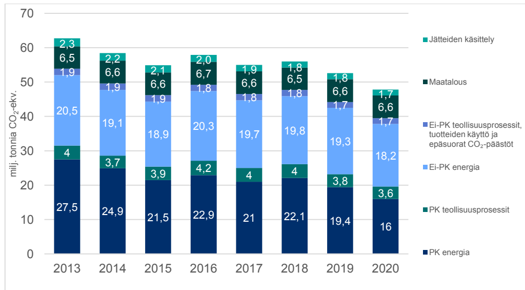
Kuva 10. Kasvihuonekaasupäästöt sektoreittain jaoteltuina päästökauppaan (PK) kuuluviin ja sen ulkopuolisiin päästöihin vuosina 2013–2020. Lähde: Tilastokeskus 2022a.
