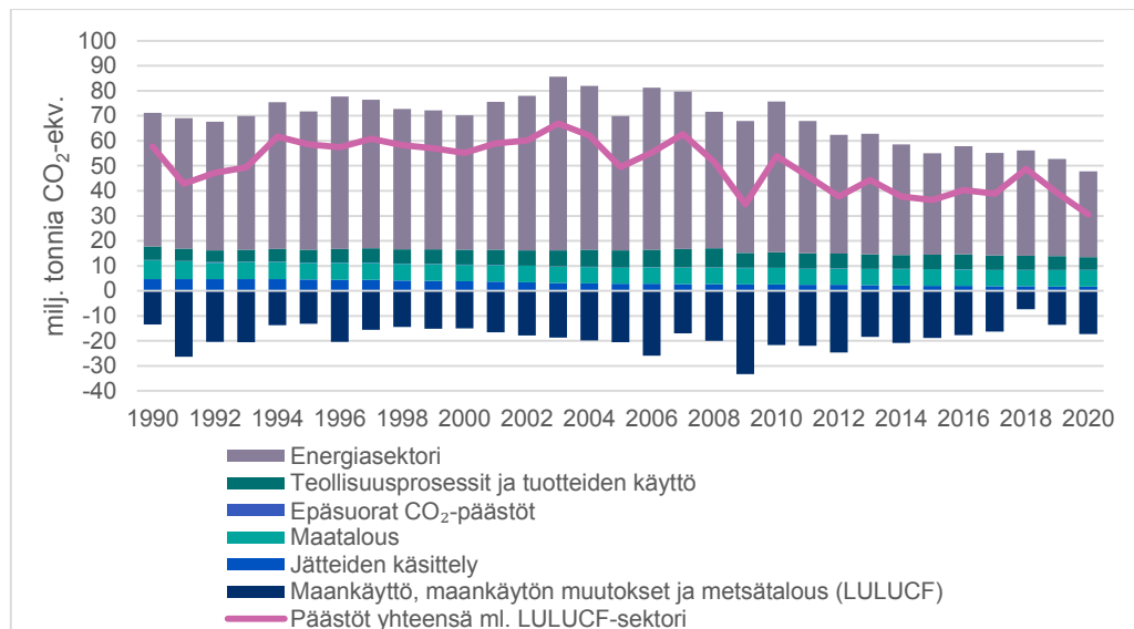
Kuva 9. Suomen kasvihuonekaasupäästöt ja -poistumat sektoreittain ja kaikkien sektoreiden summa, jossa maankäyttösektorin nettohielu on vähennetty muiden sektoreiden yhteenlasketuista päästöistä. Sektorit vastaavat Suomen kansallista kasvihuonekaasuinventaariota. Eri sektorit tai sektoreiden osat kuuluvat EU:n päästökauppa- tai taakanjakojärjestelmiin. Lähde: Tilastokeskus 2022a.
