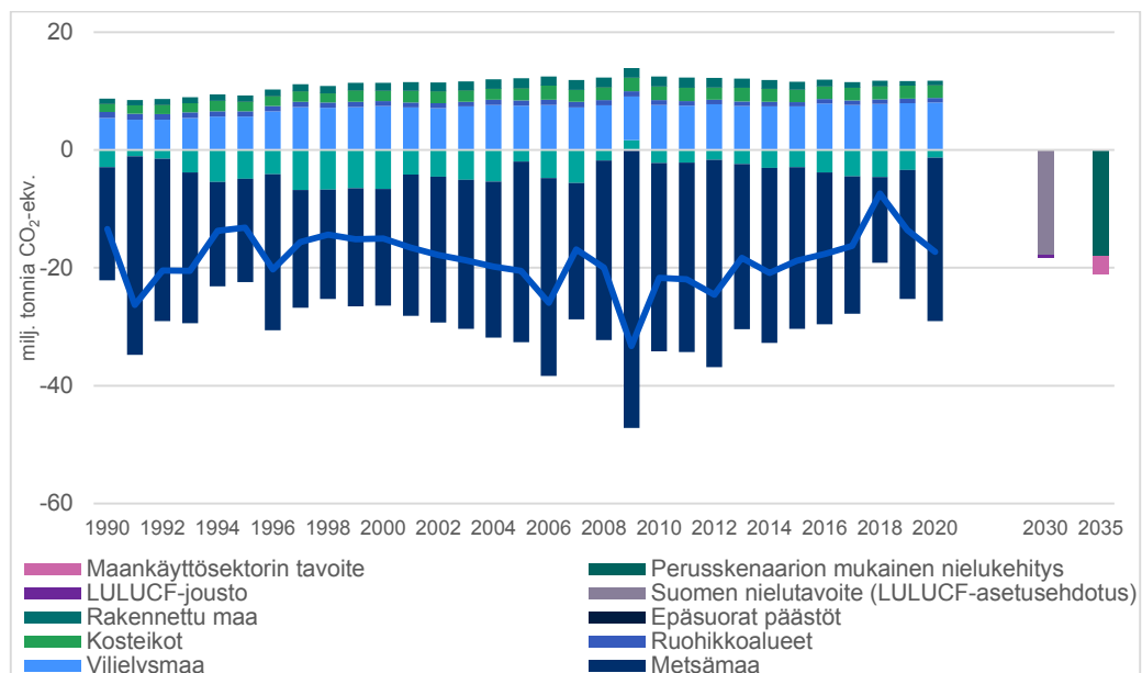
Kuva 8. Maankäyttösektorin kasvihuonekaasutaseen muutos sekä tulevat tavoitteet.
