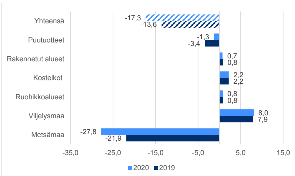
Kuva 13. Maankäyttösektorin päästöt ja poistumat maankäyttöluokittain 2019 ja 2020 (miljoonaa hiilidioksidiekvivalenttonnia) Positiivinen luku on päästöä ja negatiivinen poistumaa (nielu). Lähde: Luonnonvarakeskus 2022.
