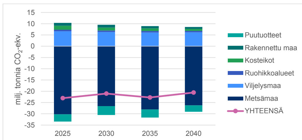
Kuva 18. Maankäyttösektorin päästöt päästöluokittain MISU-politiikkaskenaariossa, miljoonaa hiilidioksidiekvivalenttitonnia. Lähde: Luonnonvarakeskus 2022.
